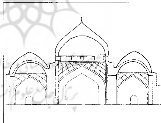
ت ۳. (راست) مقطع شرقی غربی هسته جنوبی مسجد، مأخذ: اداره کل حفاظت آثار تاریخی ارمنستان
