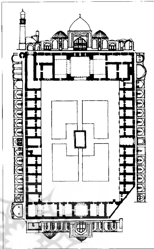
ت ۱. (راست) نقشه عمومی و نماهای صحن مسجد کبود اهروان، مأخذ: اداره کل حفاظت آثار تاریخی ارمنستان
