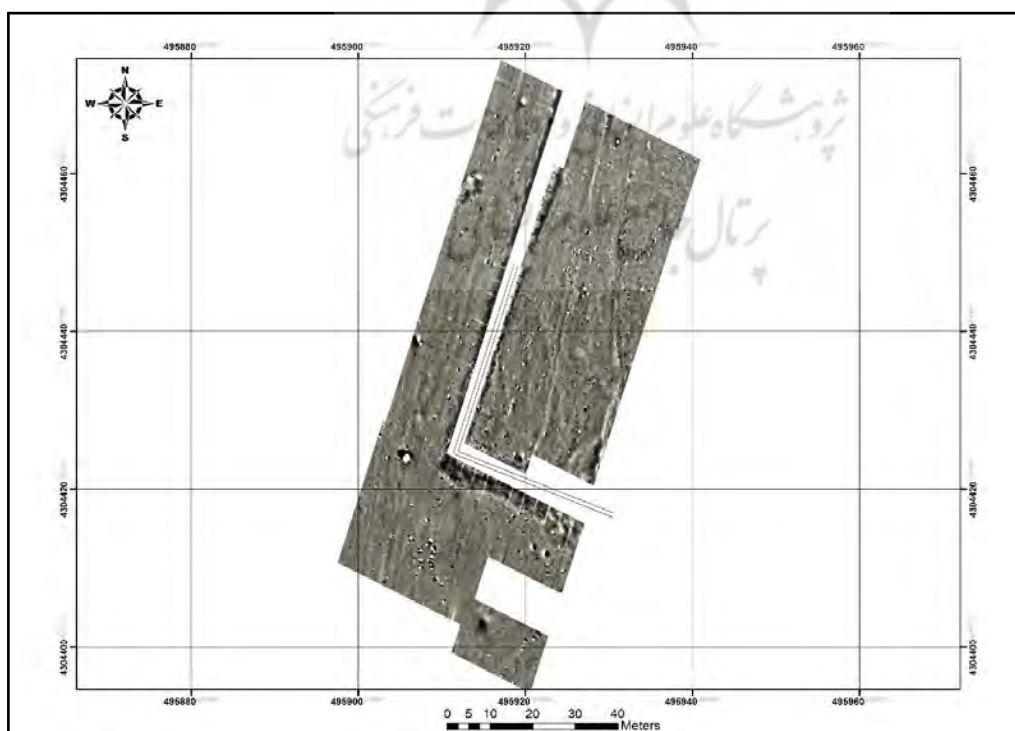
تصویر ۷. نقشه مغناطیسی محوطه مسکونی و قسمت شرقی قلعه بسنام (نگارندگان، ۱۳۹۷).
