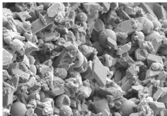
شکل ۴) تصویر میکروسکوپی از دیوار بتنی با میکروکپسول‌های PCM [22]
