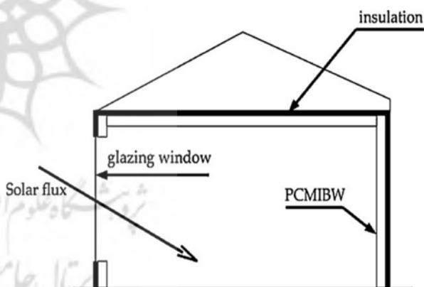
شکل ۳) کاربرد و عملکرد مواد تغییر فاز دهنده دیواری [22]
