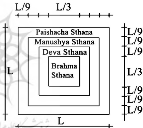
شکل (۳) الگوی هندسی معماری واستو [43]
