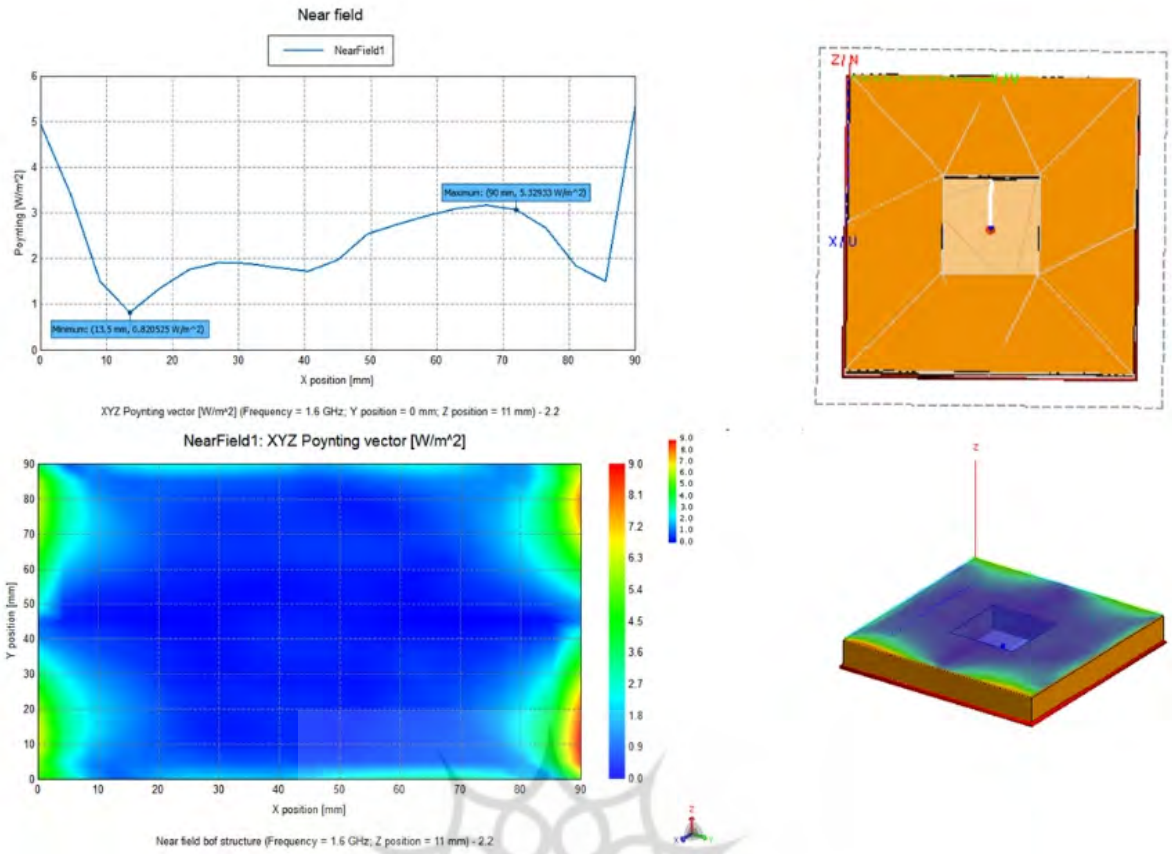
شکل ۸) دیاگرام شدت میدان‌های الکترومغناطیسی در مدل شماره دو
