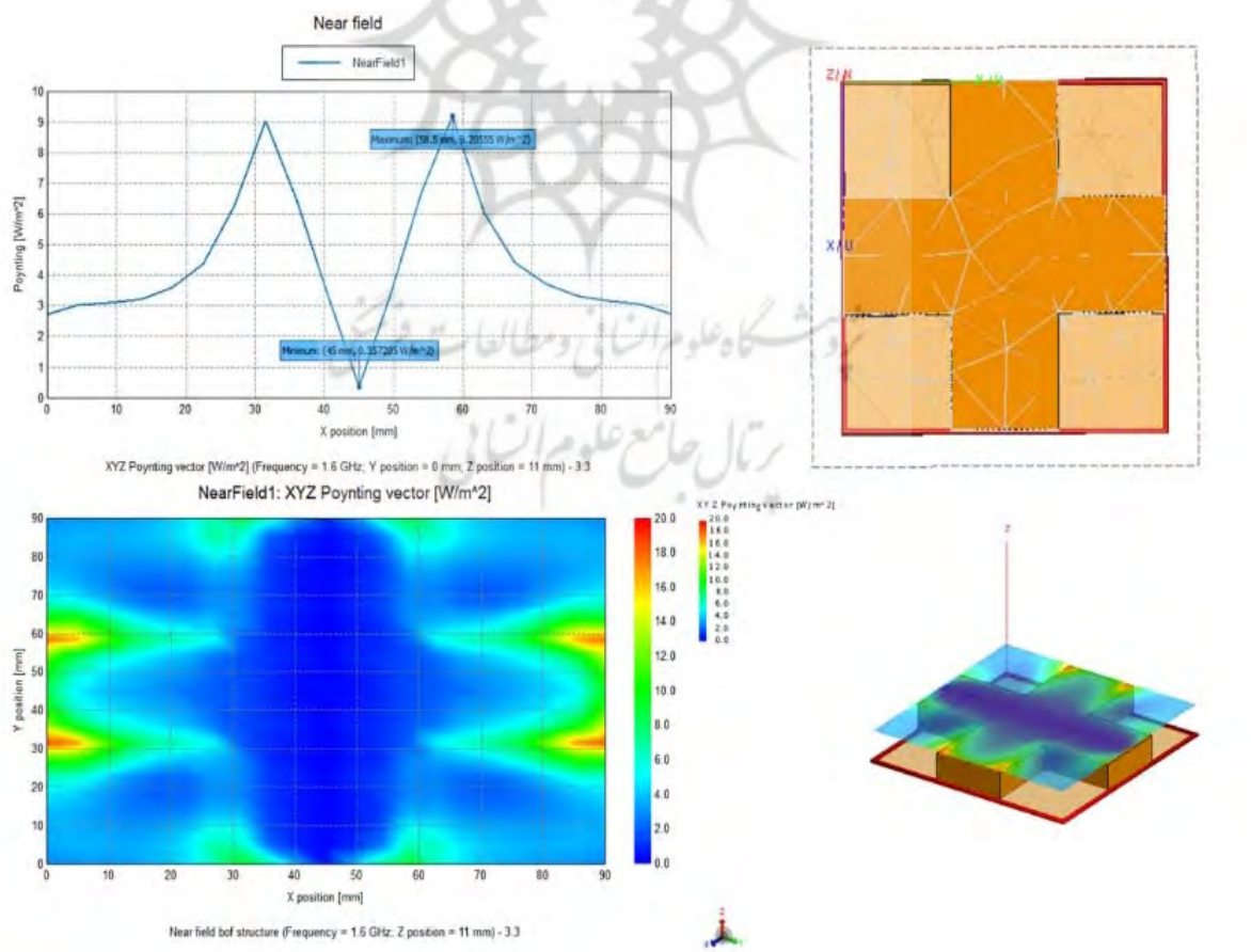
شکل ۹) دیاگرام شدت میدان‌های الکترومغناطیسی در مدل شماره سه
