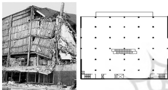
شکل ۱) تخریب ساختمان جی.سی.بنی در زلزله ۱۹۶۴ آلاسکا در اثر پیچش ناشی از چیدمان دیوارها [1]
