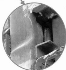
شکل ۱۳) شکست ستون به دلیل سوراخ‌کردن آن برای عبور تیر؛ زلزله ۱۳۸۲ بم [26]
