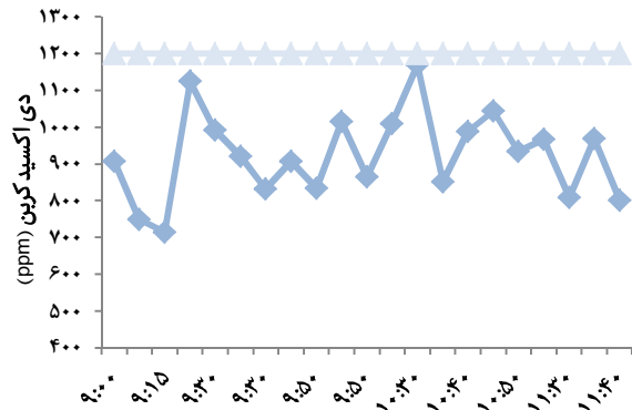
نمودار ۲) ساختمان شماره ۱ با میانگین مقدار دی‌اکسیدکربن ۹۲۳/۶ppm
