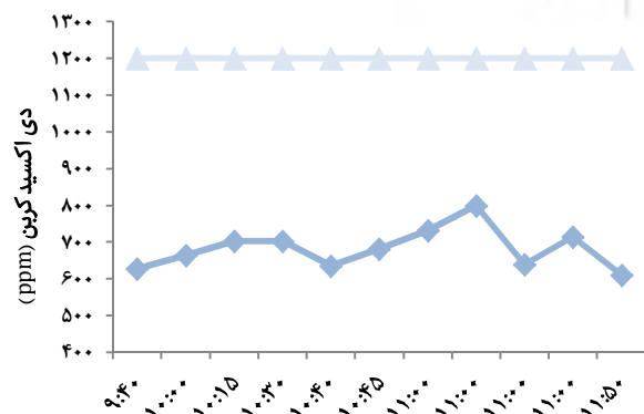
نمودار ۴) ساختمان شماره ۳ با میانگین مقدار دی‌اکسیدکربن ۶۸۲/۹ppm
