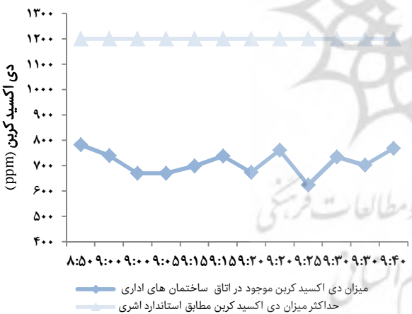
نمودار ۱۱) ساختمان شماره ۱۰ با میانگین مقدار دی‌اکسیدکربن ۷۱۳ppm
