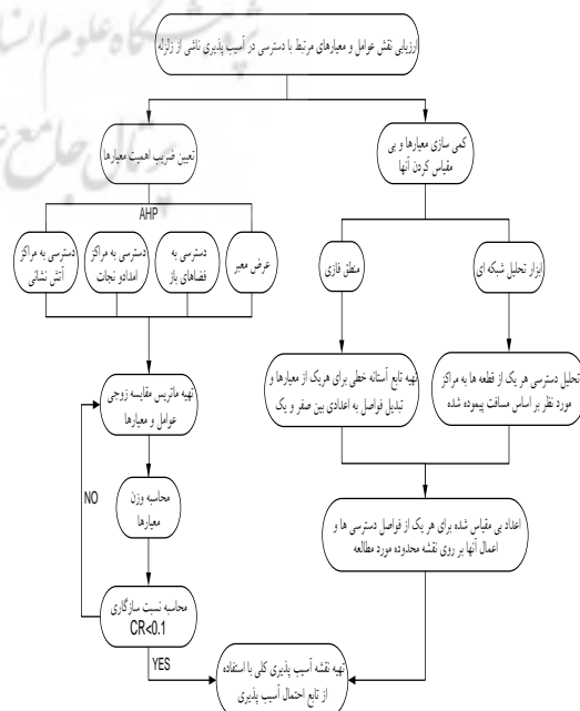
شکل ۲: مدل پیشنهادی برای ارزیابی آسیب پذیری ناشی از عامل دسترسی
