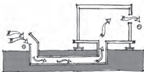
شکل ۱۲. بادخور در فاصله کمی از ساختمان قرار گرفته است هوا از مجرای لوله‌های زیرزمینی تامین می‌شود و هوارا پیش‌خنک می‌کند. منبع: محمودی، ۱۳۸۸
