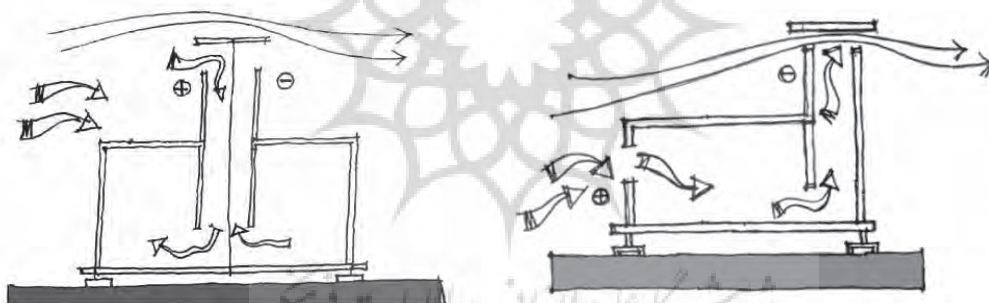
شکل ۹. در ساختار بادگیرها عضو ورودی و خروجی با هم در یک مجموعه تعبیه شده است. منبع: محمودی، ۱۳۸۸
