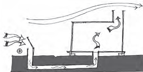
شکل ۱۰. بادخورها هوا را از طریق لوله‌های زیرزمینی تأمین می‌کنند و هوا از طریق بادخوان خارج می‌شود. منبع: محمودی، ۱۳۸۸
