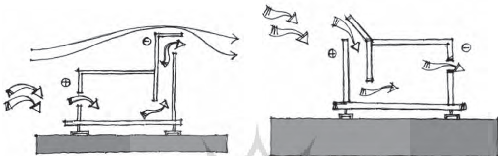
شکل ۷. بادخوان زانویی، منبع: محمودی، ۱۳۸۸
