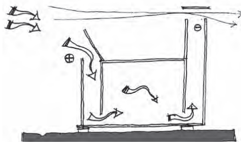
شکل ۱۱. ترکیب بادخور (به عنوان ورودی) و بادخوان (به عنوان خروجی). منبع: محمودی، ۱۳۸۸
