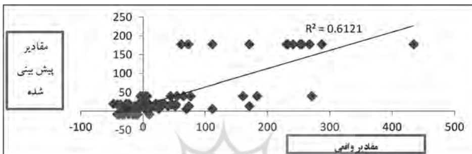
شکل شماره ۱. همبستگی بین مشاهدات با مقادیر پیش‌بینی‌شده (متغیرهای کلان اقتصادی با بازده سهام شرکت‌های شستا) با روش شبکه فازی عصبی تطبیقی
