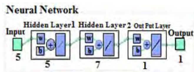
شکل شماره (۵): شبکه عصبی مورد استفاده
