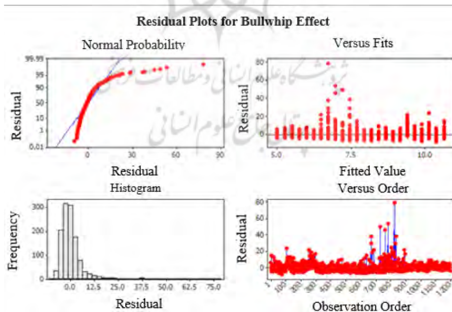
شکل شماره (۹): بررسی فرضیات واریانس
