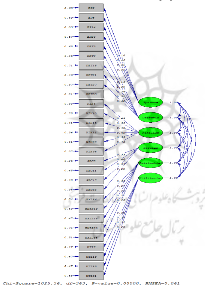
دیاگرام شماره ۱ مدل نظری تحلیل عاملی تأییدی
