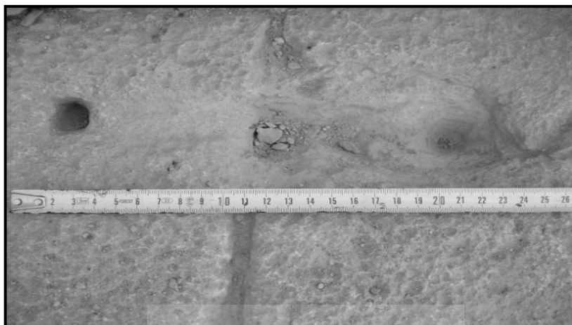
تصویر شماره ۱۴: نمایی از نوع دوم بست‌های بکار رفته در پلکان آرامگاه گوردختر بزپر که یک سر آنها به صورت مدور و سر دیگر به صورت مستطیل شکل می‌باشد.
