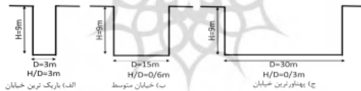
شکل ۱۹- مقطع عرضی خیابان طراحی شده در سایت
