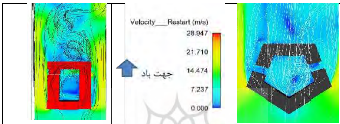
شکل ۷: شبیه‌سازی جریان باد در مدل‌های بسته‌ای از حیاط مرکزی. منبع: (نگارندگان برگرفته از نرم‌افزار ۲d flow)
