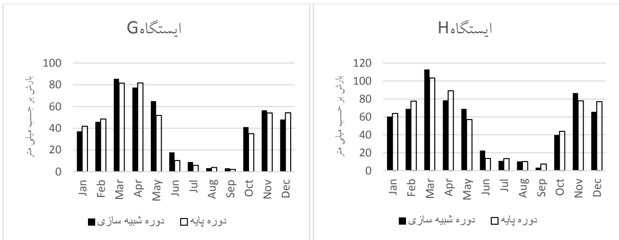
شکل ۵. تغییرات ماهانه بارش در دوره ۲۰۱۶-۲۰۲۹ نسبت به دوره پایه
