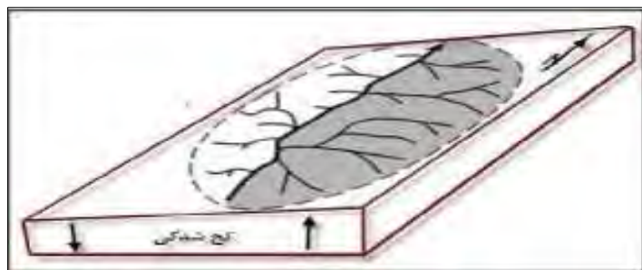
شکل ۶. بلوک دیاگرام یک حوضه‌ی زهکشی متأثر از حرکات فرایشی (تکتونیک). مأخذ: مقصودی و همکاران، ۱۳۸۸
