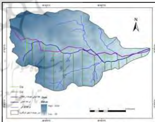
شکل ۱۴. ارزیابی شاخص (T) در حوضه کرگانرود. مأخذ: نویسندگان، ۱۳۹۵
