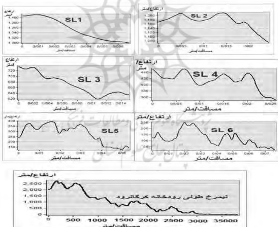
شکل ۹. نیمرخ طولی رودخانه‌ی کرگانرود به همراه مقادیر SL. مأخذ: نویسندگان، ۱۳۹۵
