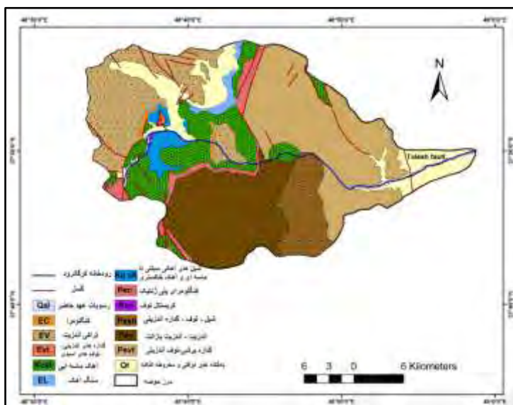
شکل ۲. نقشه زمین‌شناسی حوضه آبخیز کرگانرود مأخذ: نویسندگان، ۱۳۹۵
