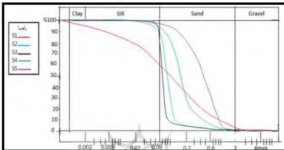
شکل ۶: منحنی گرانولومتری رسوبات پلایای سبزوآر
