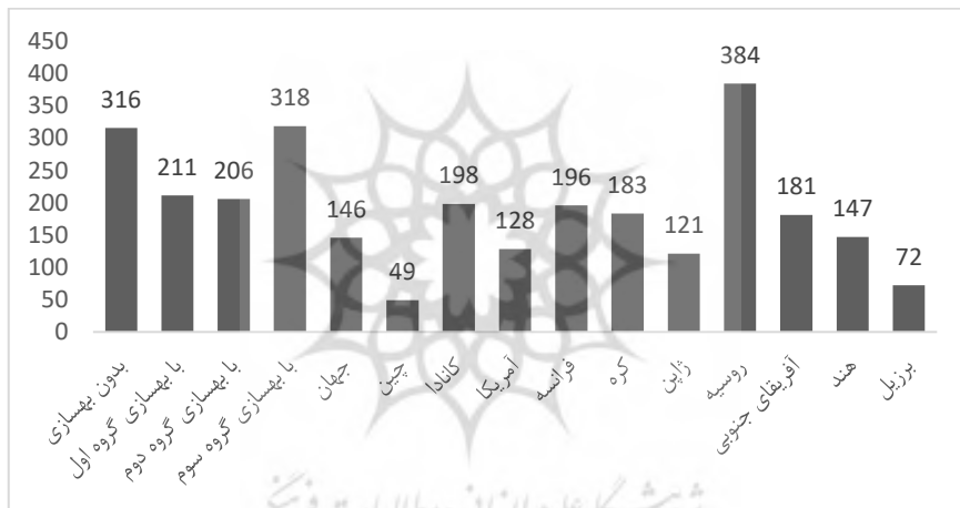
نمودار ۴. مقایسه بین‌المللی متوسط مصرف انرژی به ازای هر متر مربع خانه‌های مسکونی (IEA, 2015)
