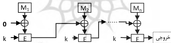
شکل (۳) ساختار مد CBC
