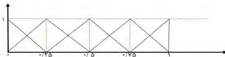
نمودار شماره (۱): اعداد فازی مثلثی معادل طیف لیکرت
