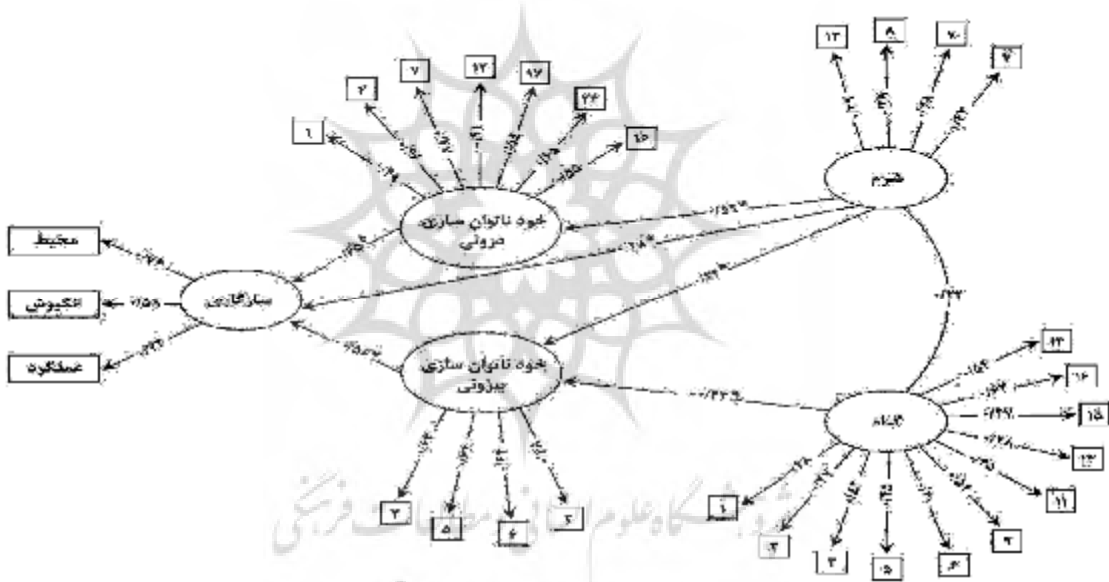
شکل 2. مدل پژوهش
