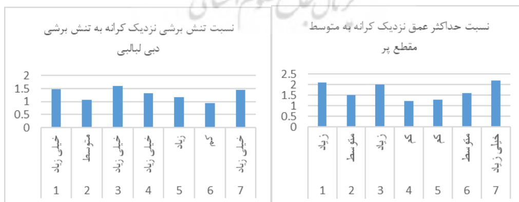
شکل (۲). نمودار تغییرات شاخص‌های NBS در مقاطع عرضی
