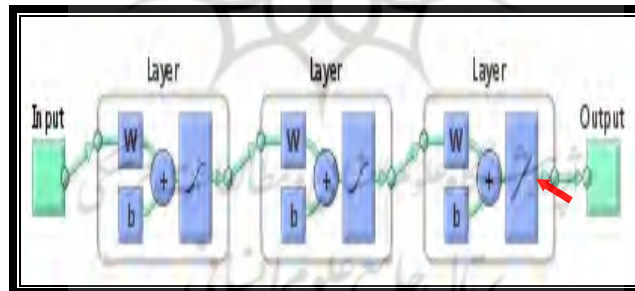
شکل (۴) شماتیک شبکه پرسپترون چندلایه طراحی شده
