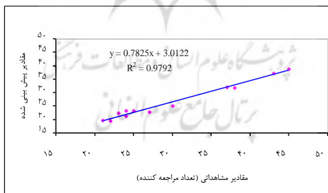
شکل (۶) رابطه رگرسیونی بین مقادیر مشاهده‌ای و پیش‌بینی شده تعداد مراجعین کننده بیماری آسم
