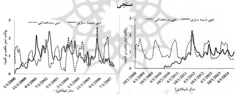
شکل (۴) شبیه‌سازی دبی حوضه نیر با مدل IHACRES: الف) دوره واسنجی ب) دوره اعتبار
