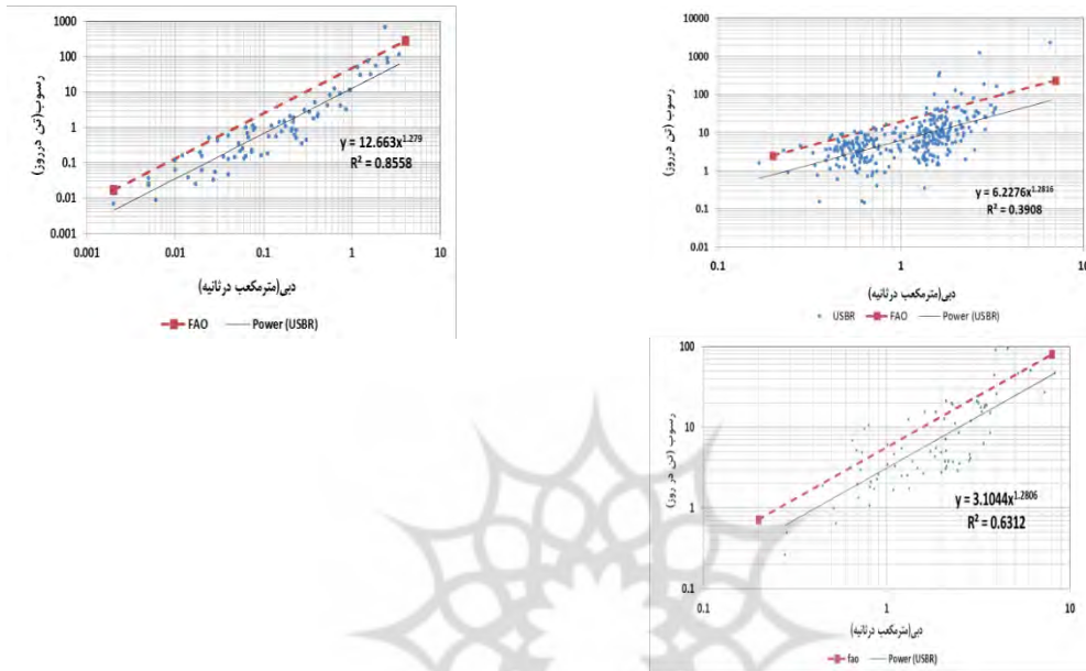
شکل (۵) نمودار همبستگی نمایی و رسوب رودخانه در حوضه‌های الف) آتشگاه، ب) عموقین، پ) کوزه توپراقی، ت) نوران، ث) نیر، ج) باروق و چ) یامچی
