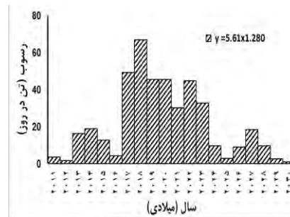
شکل (۶) مقادیر میانگین رسوب برای دوره آتی (۲۰۳۰-۲۰۱۱) در حوضه‌های الف) آتشگاه، ب) عموقین، پ) کوزه توپراقی، ت) نوران، ث) نیر، ج) باروق و چ) یامچی
