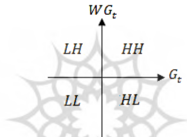
شکل ۱. نمودار موران
