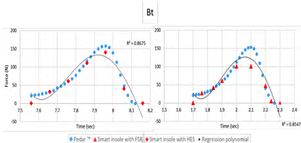
شکل ۱۵- نتایج همبستگی و تطبیق Bt دو نمودار حاصل از پدار و کفی اثر هال و کفی FSR با ضریب رگرسیون ۰/۸۷ و ۰/۸۵
