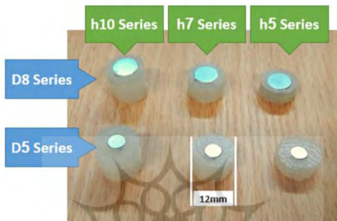
شکل ۴- سنسورهای اثر هال با ارتفاع و قطر آهن‌ربای مختلف
