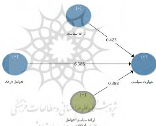
شکل ۵: مدل ساختاری در حالت اعداد معناداری تعدیلی
