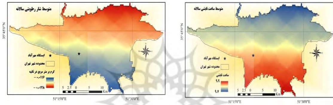
شکل ۳. الگوی فضایی متوسط سالانه تابش خورشید (راست) و شار لحظه‌ای رطوبت (چپ)
