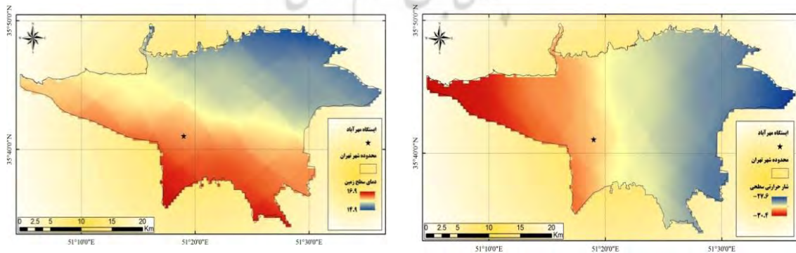
شکل ۴. الگوی فضایی متوسط سالانه شار لحظه‌ای گرمای محسوس (راست) و دمای سطحی (چپ)
