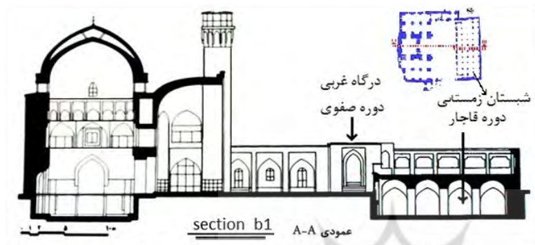
شکل ۱۰. برش عمودی A-A مسجد جامع، مأخذ میراث فرهنگی لرستان
