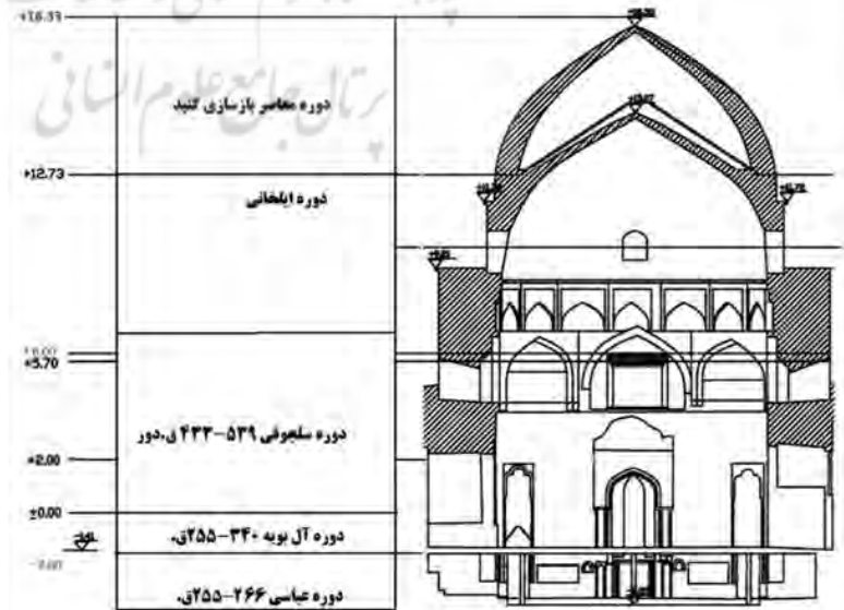
شکل ۷. برش مسجد جامع بروجرد و مقاطع تاریخی آن (مأخذ آرشینو میراث فرهنگی لرستان، تغییر از نگارنده)
