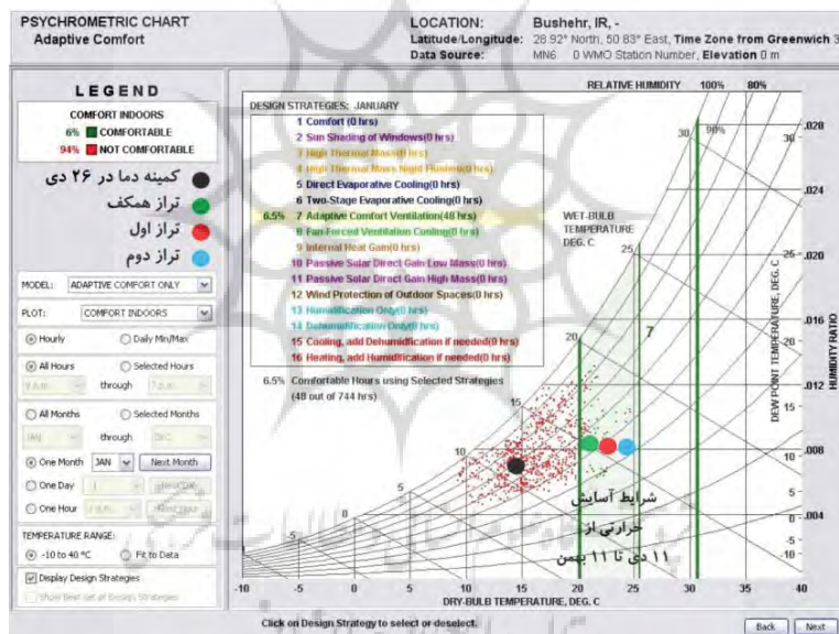
تصویر ۱۲. وضعیت سردترین ساعت شب در بیرون از ساختمان و در بهترین فضا از هر تراز در همان ساعت در دی (ماخذ: نگارنده، از نرم‌افزار کلاسیک کانسالنت)
