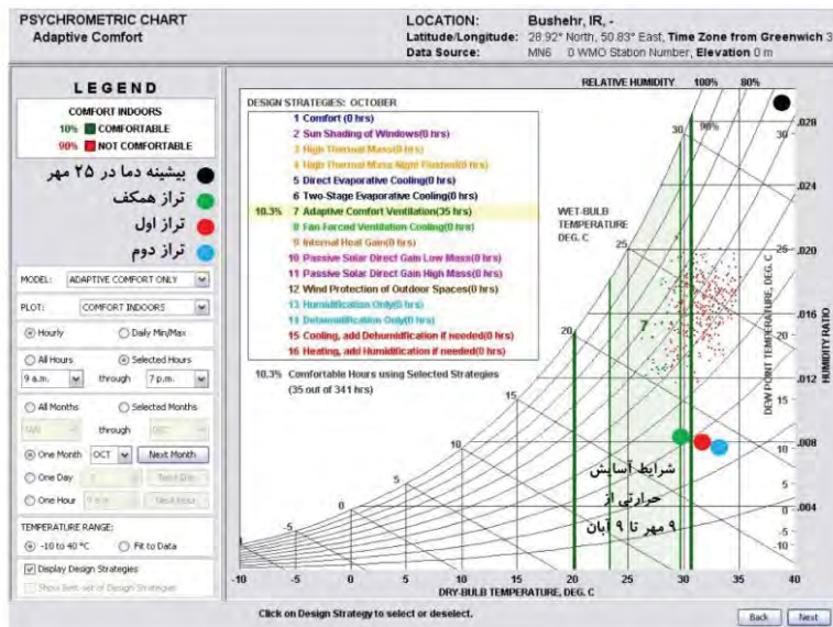
تصویر ۱۱. وضعیت گرمترین ساعت روز در بیرون از ساختمان و در بهترین فضا از هر تراز در همان ساعت در مهر (ماخذ: نگارنده، از نرم‌افزار کلاسیک کانسالنت)
