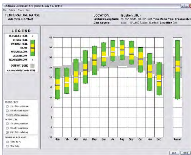
تصویر ۶. نمودار دما در مقایسه با شرایط آسایش با مدل آسایش تطبیقی (ماخذ: نگارنده، از نرم‌افزار کلاسیک کانسالنت)
