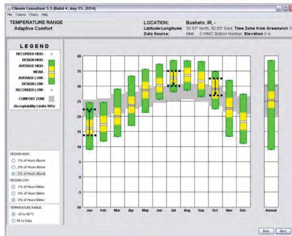
تصویر ۹. نمایش میزان بیشترین کاهش دما در سه ماه مورد بررسی (ماخذ: نگارنده، از نرم افزار کلاسیک کانسالنت)
