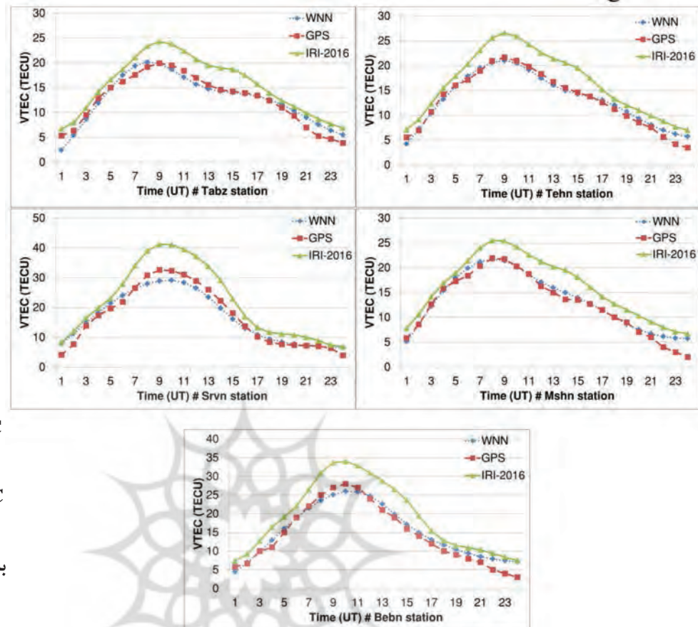
نگاره ۶: مقایسه مقادیر VTEC برآورد شده در ۵ ایستگاه آزمون با مقادیر VTEC حاصل از GPS و مدل مرجع جهانی ۲۰۱۶ با تعداد ۱۵ ایستگاه آزمون
