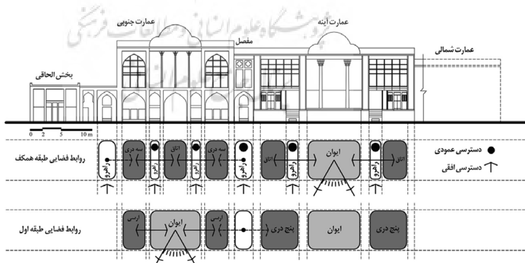
تصویر ۸: روابط فضایی پیشنهادی فضاهای داخلی در مجموعه کاخ آینه
