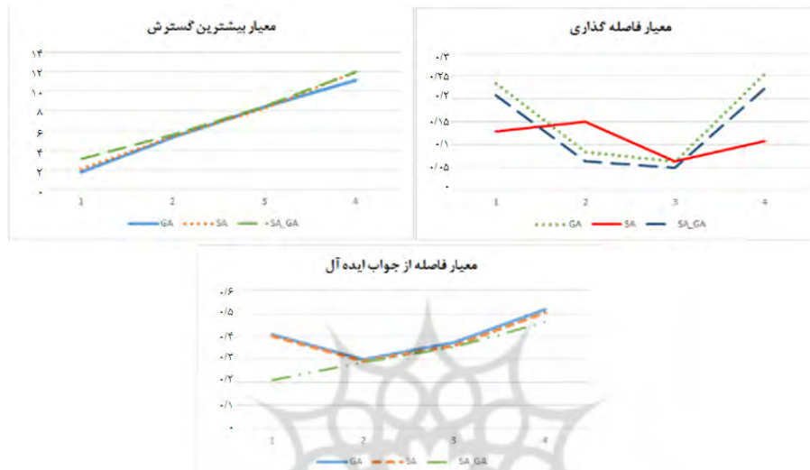
شکل ۱۲. خلاصه‌ای از عملکرد الگوریتم‌های فراابتکاری از منظر معیارهای پارتو بر اساس ۴ مسئله نمونه‌ای بزرگ
