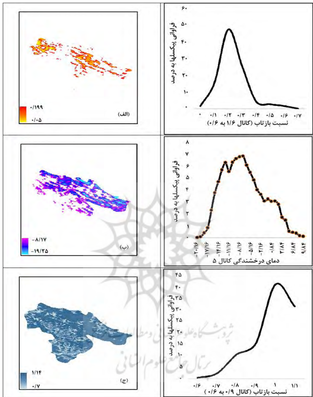
شکل ۶. الف) نسبت کانال 3a به کانال 1؛ ب) دمای درخشندگی کانال 5؛ ج) نسبت بازتاب کانال مادون قرمز نزدیک (0/9) به مرئی (0/6) در روز 12 ژانویه 2008 ساعت 7:33 با داده‌های NOAA17
