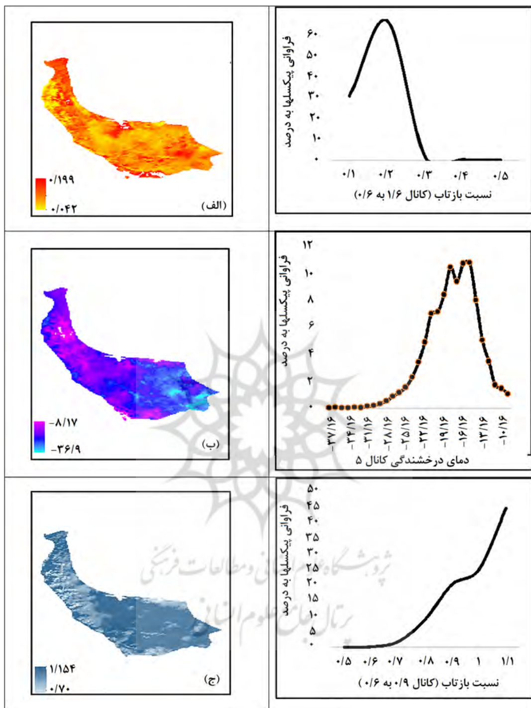
شکل ۵. الف) نسبت کانال ۳a به کانال ۱؛ ب) دمای درخشندگی کانال؛ ج) نسبت بازتاب کانال مادون قرمز نزدیک (۰/۹) به مرئی (۰/۶) در روز ۱۲ ژانویه ۲۰۰۸ ساعت ۷:۳۳ با داده‌های NOAA17
