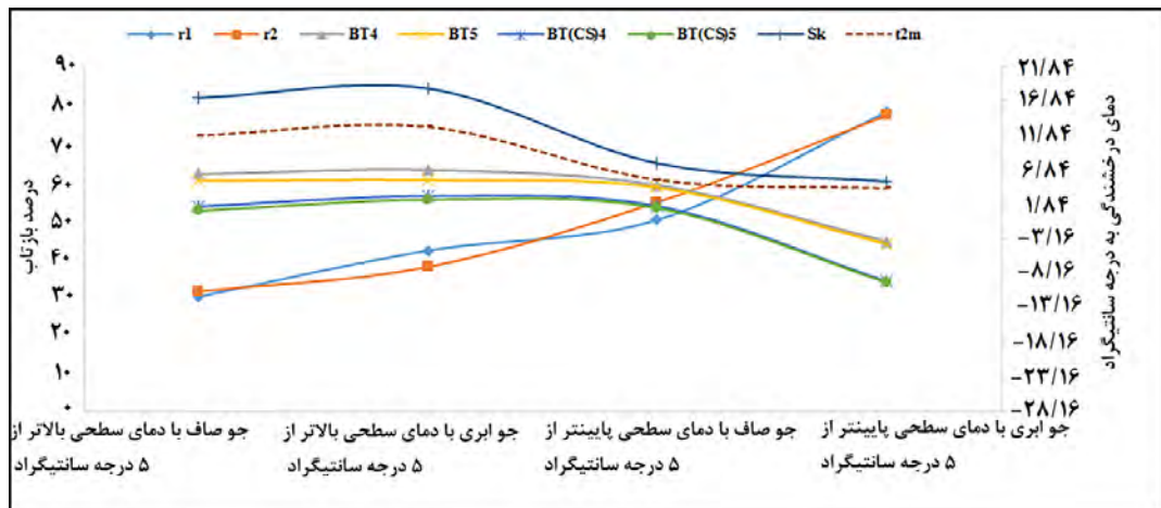
شکل ۸. میانگین بازتاب در کانال ۱ و ۲، دمای درخشندگی کانال ۴ و ۵، دمای درخشندگی جو بدون ابر در کانال ۴ و ۵، که به ترتیب با نمادهای 5, BT(CS)5, BT(CS)4, BT5, BT4, r2, و r1 برای استان کهگیلویه و بویراحمد نمایش داده شده است
