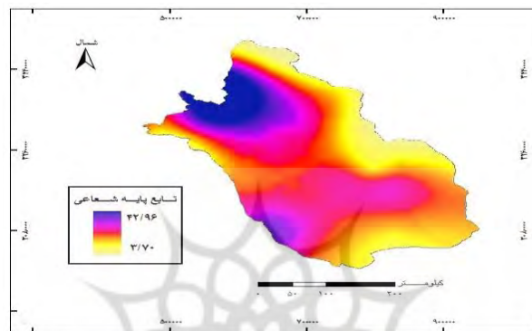
شکل ۵. نقشه پهنه بندی شاخص فرساینده با روش RBF
