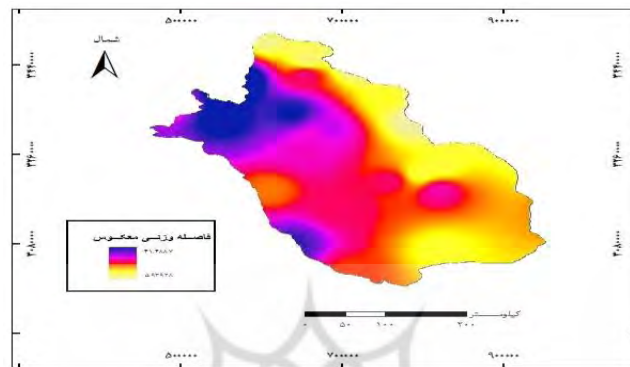
شکل ۲. نقشه پهنه‌بندی شاخص فورنیبه با روش IDW
