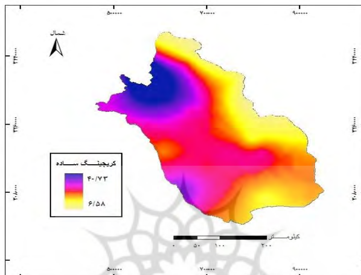
شکل ۸. مدل چهاروجهی از روش کریجینگ ساده
