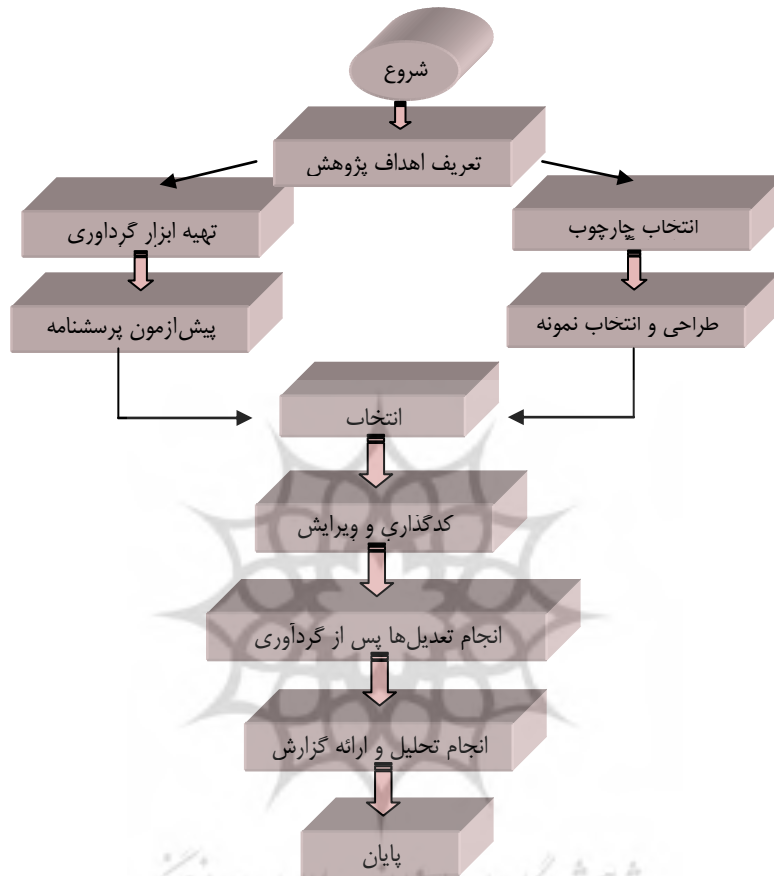
شکل ۱. الگوریتم نمونه‌گیری
