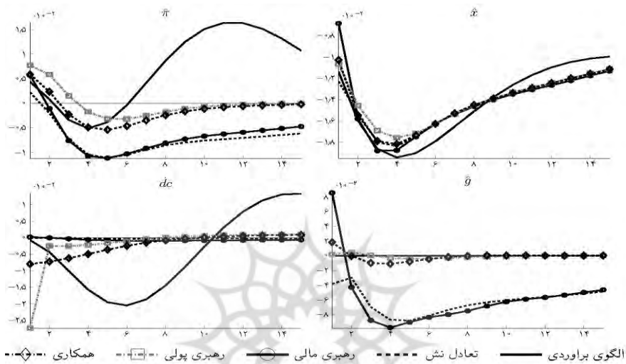
شکل ۵. توابع واکنش آنی نسبت به تکانه \varepsilon
