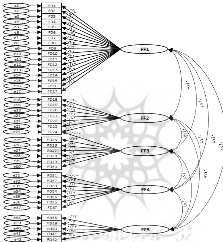
شکل ۱. مدل عاملی پرسشنامه FDE و بارهای عاملی استاندارد در کل نمونه
