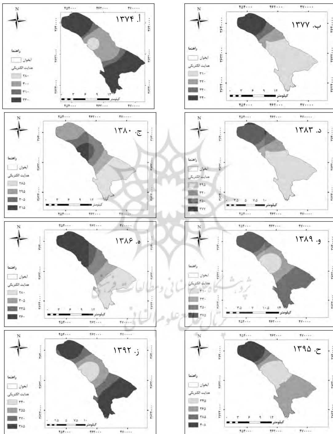
شکل ۳: توزیع شوری آب (بر حسب میکروزیمنس بر سانتی متر) در آبخوان چادگان در سال های متعدد (أ تا ح) ۱۳۹۵ (منبع: سازمان آب منطقه ای اصفهان، ۱۳۹۵)
