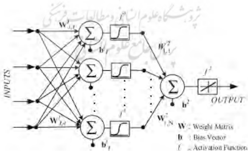
شکل ۱: ساختار شبکه عصبی پرسپترون چندلایه
