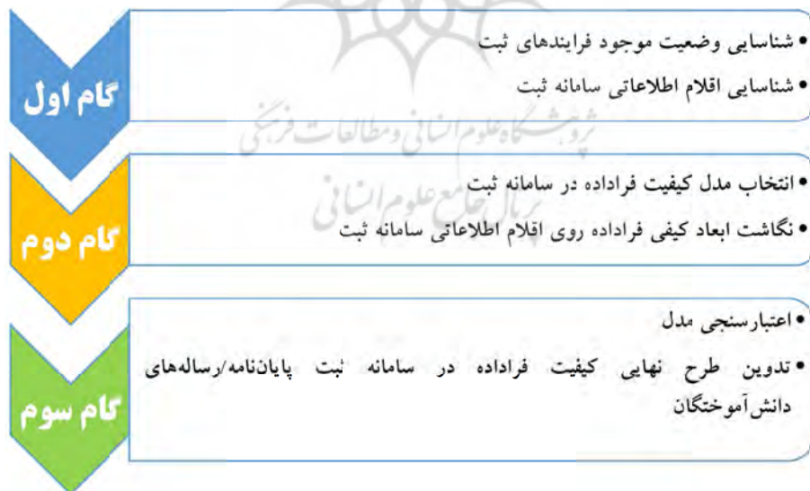
شکل ۴. گام‌های پژوهش
