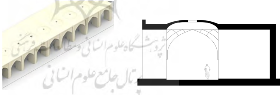
تصویر ۱: برش از بازارهای اطراف در مرحله اول شکل‌گیری میدان نقش جهان
