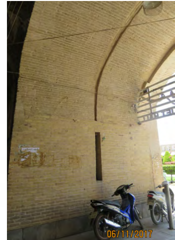
تصویر ۶: دهانه شاهد به عمق ۲۰ سانتی‌متر بین جرز اول و دوم در محل توسعه بدنه میدان در یکی از دهانه‌های بدنه شرقی
