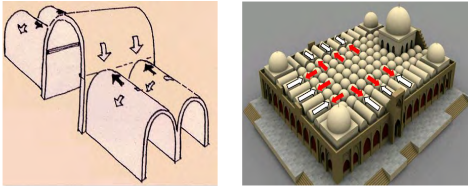
شکل ۷. کاربرد اصل تقابل نیرو در پوشش مسجد جامع گلبرگه (نگارنده، ۱۳۹۶) (راست)
