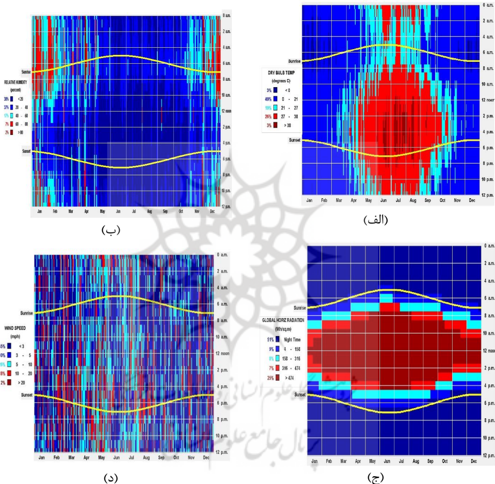
شکل (۱). بررسی زمانی شرایط آسایش حرارتی قبل و بعد از طلوع آفتاب در یزد (الف تا د) (منبع: نگارندگان، ۱۳۹۷)
