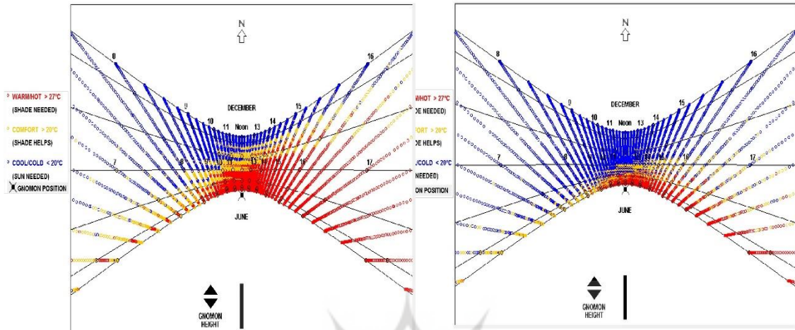
شکل (۵). حرکت سایه خورشید دوره (تابستان-پاییز) (منبع: نگارندگان، ۱۳۹۷)
