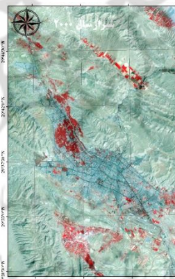
شکل (۱). منطقه مورد مطالعه، شیراز
