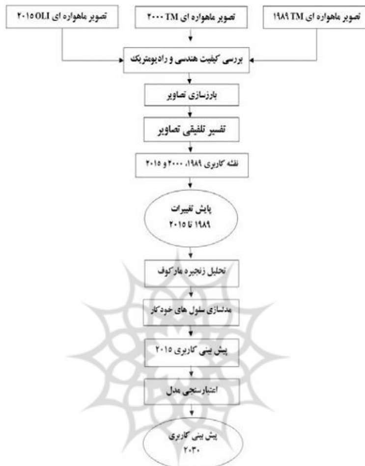
شکل (۵). چارچوب مفهومی پایش و پیش بینی تغییرات کاربری و پوشش زمین (دزکام و همکاران، ۱۳۹۴)
