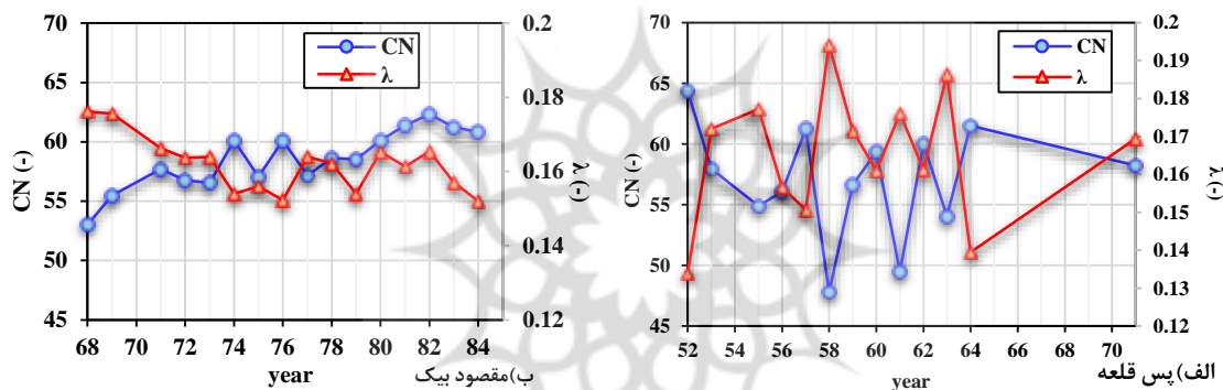
شکل ۳ روند تغییرات سالانه پارامترهای (CN)، ( \lambda ) دو حوضه آبریز پس‌قلعه (الف) و مقصودبیک (ب) که توسط مدل SCS
