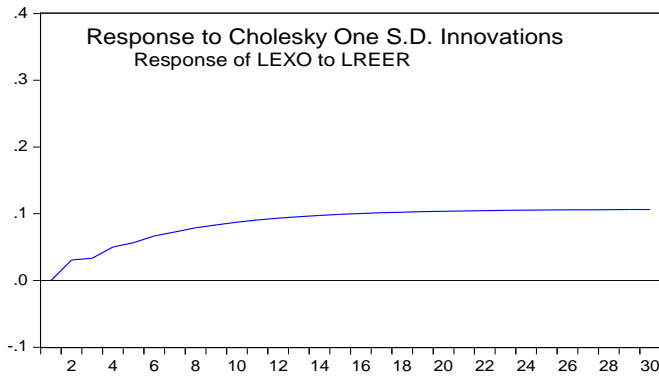
تصویر ۳. تابع عکس العمل برون گرایی اقتصاد نسبت به شوک مثبت (یک انحراف معیار) در نرخ ارز
