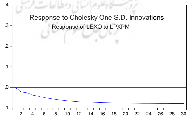
تصویر ۴. تابع عکس العمل برون گرایی اقتصاد نسبت به شوک مثبت (یک انحراف معیار) در نسبت قیمت کالاهای صادراتی به وارداتی
