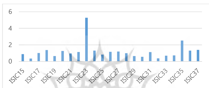
نمودار ۱ تغییر شدت انرژی بخش صنعت به تفکیک کدهای ISIC ۲ طی دوره ۱۳۸۳-۱۳۹۳
