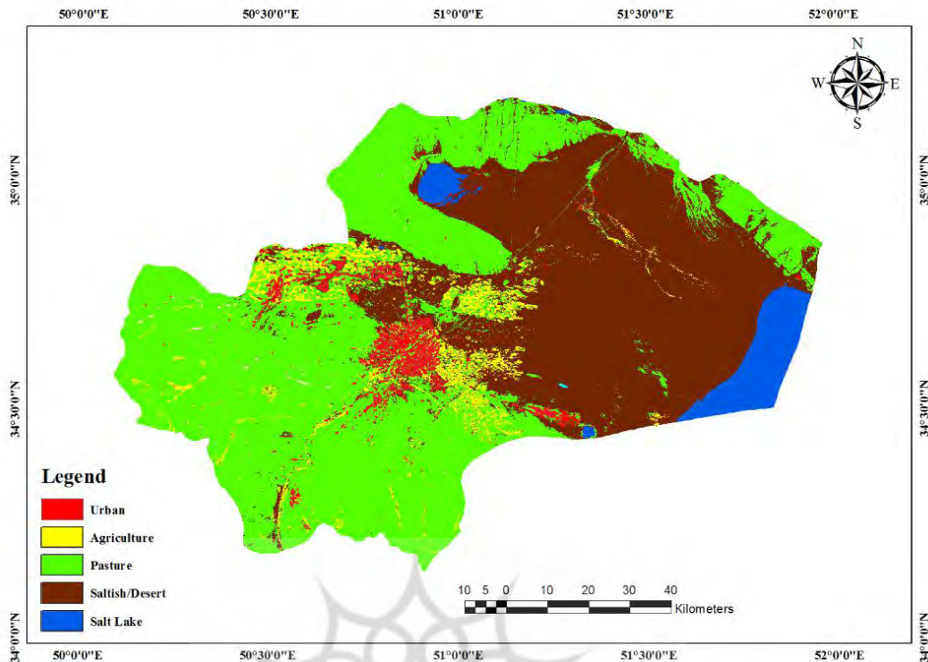
شکل ۶. کاربری اراضی پیش‌بینی شده برای ۱۰ سال آینده (سال ۱۴۰۵) منطقه مورد مطالعه با استفاده از زنجیره مارکوف (منبع: نویسنندگان، ۱۳۹۵)
