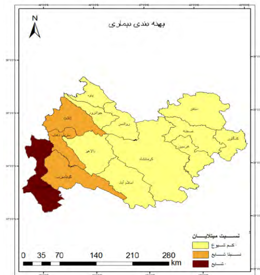
شکل - ۴: بهنه بندی بیماری سالک
