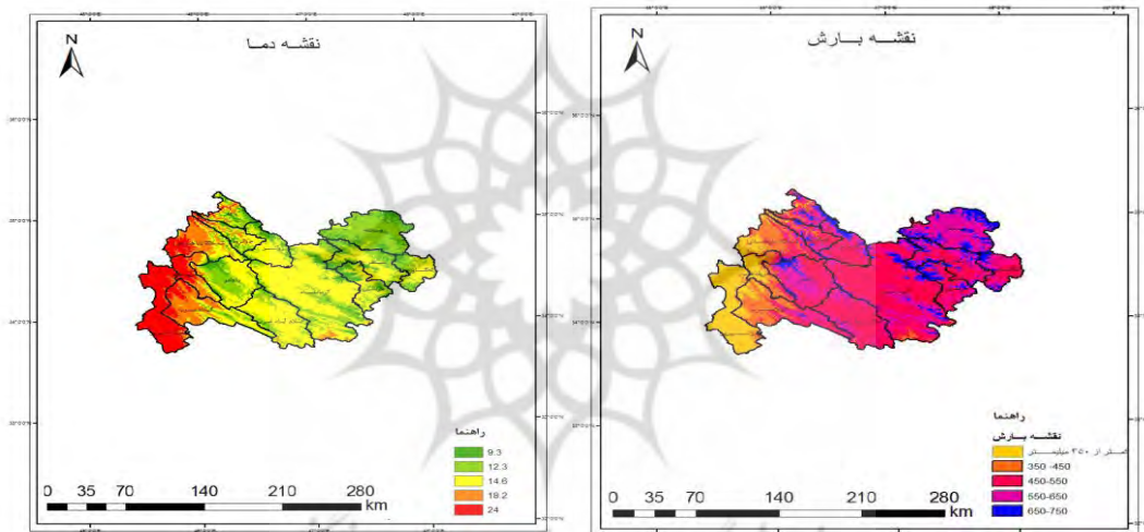
شکل - ۵: نقشه دما شکل - ۶: نقشه بارش
